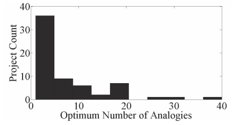
(a) Cocomo81
